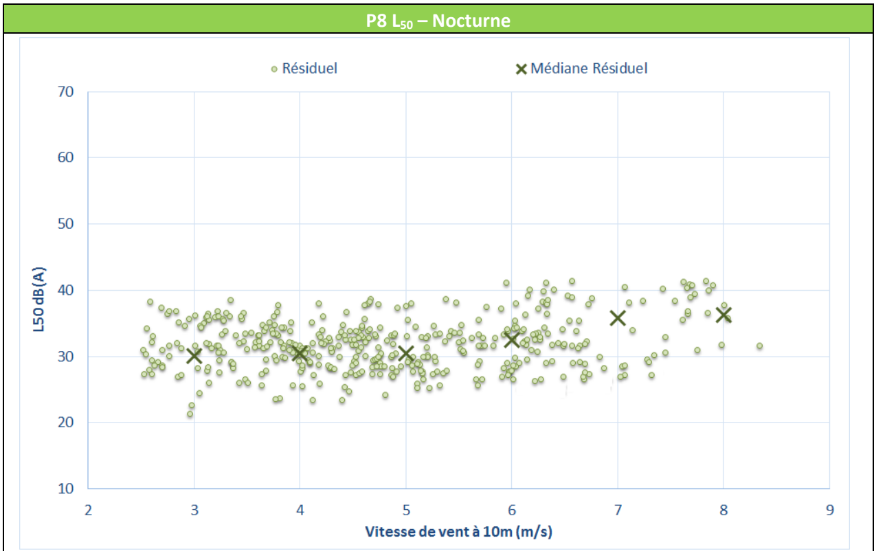
Figure 29 : Bruit en fonction de la vitesse de vent au point P8 – Mesures estivales
