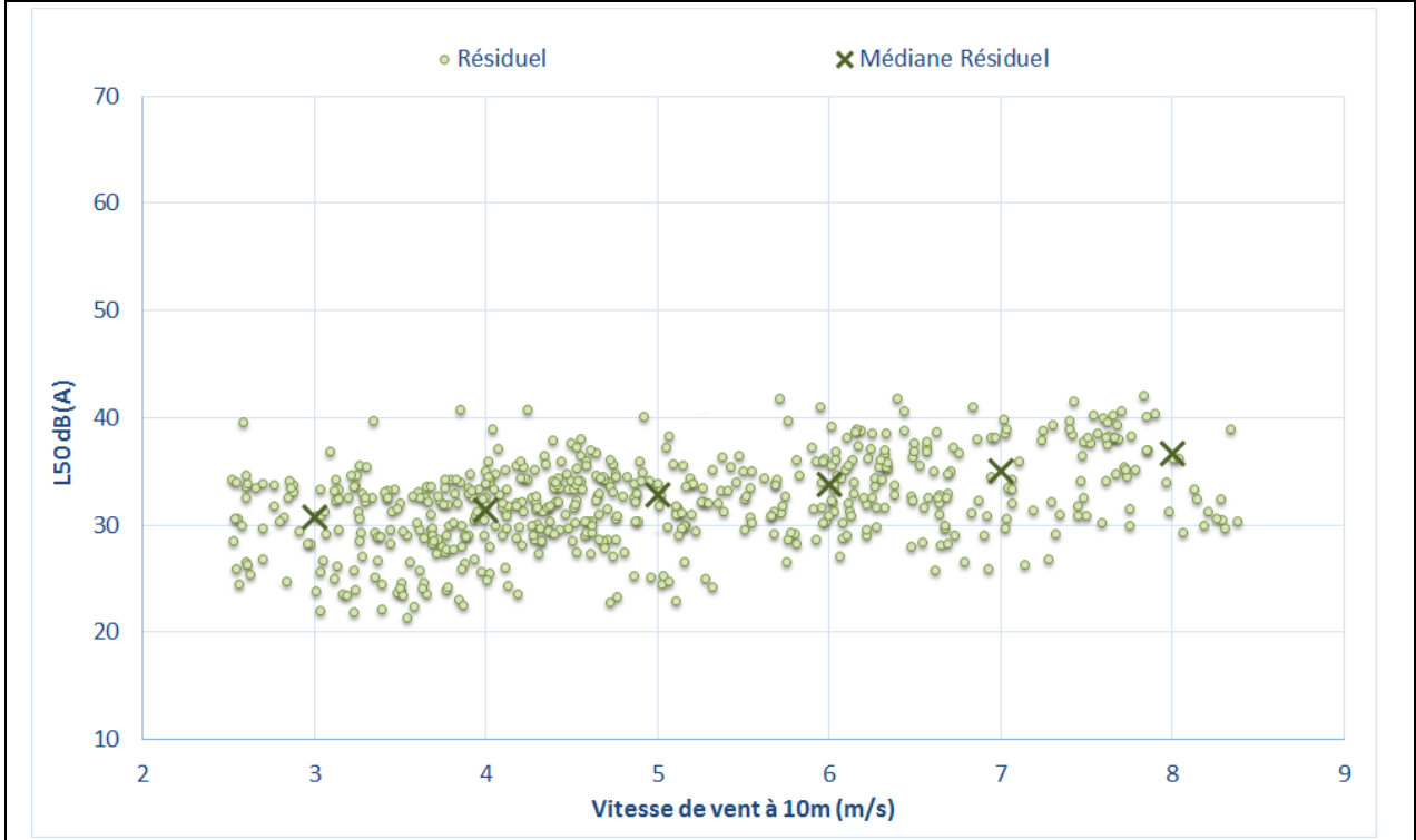
Figure 27 : Bruit en fonction de la vitesse de vent au point P6 – Mesures estivales
