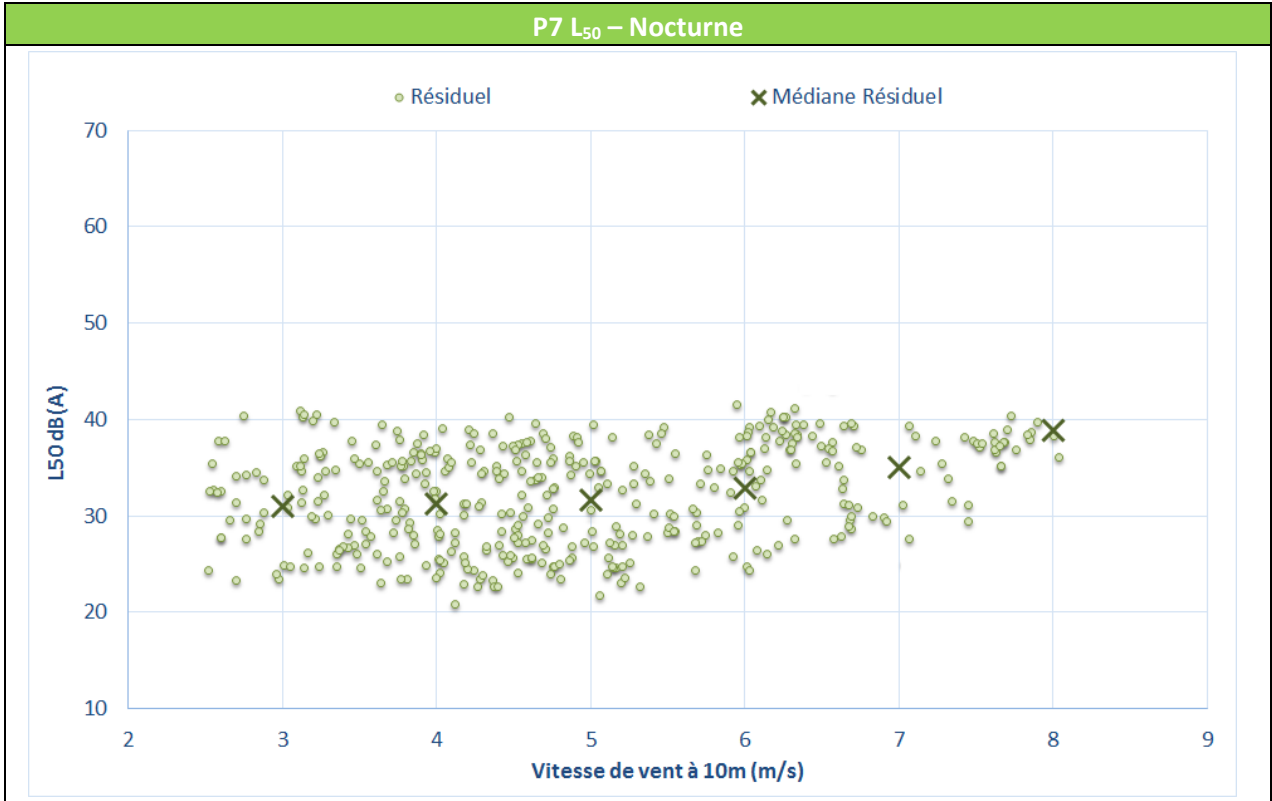
Figure 28 : Bruit en fonction de la vitesse de vent au point P7 – Mesures estivales
