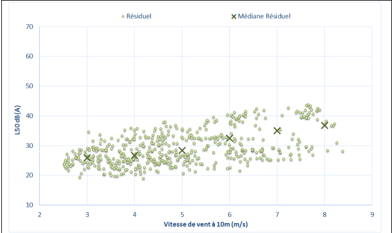
Figure 30 : Bruit en fonction de la vitesse de vent au point P9 – Mesures estivales
