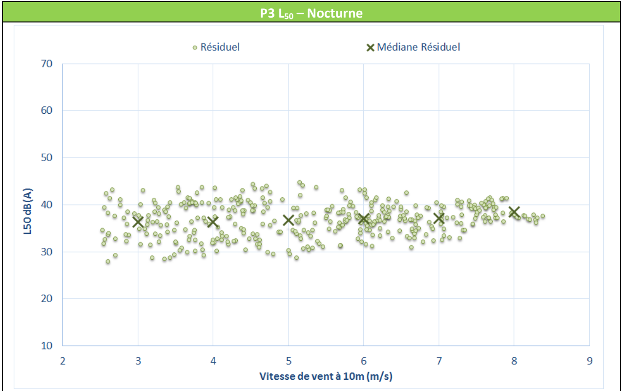
Figure 24 : Bruit en fonction de la vitesse de vent au point P3 – Mesures estivales
