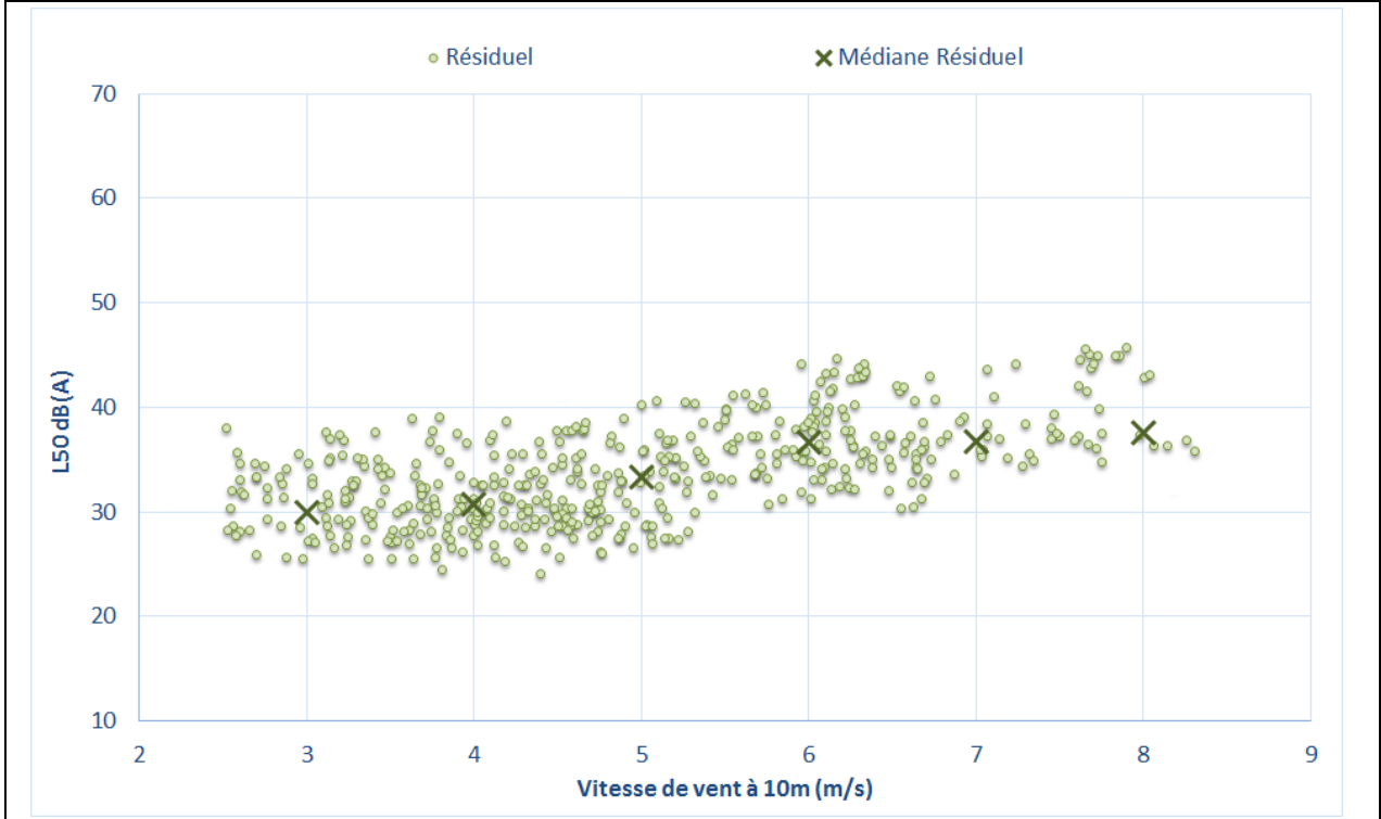
Figure 23 : Bruit en fonction de la vitesse de vent au point P1 – Mesures estivales
