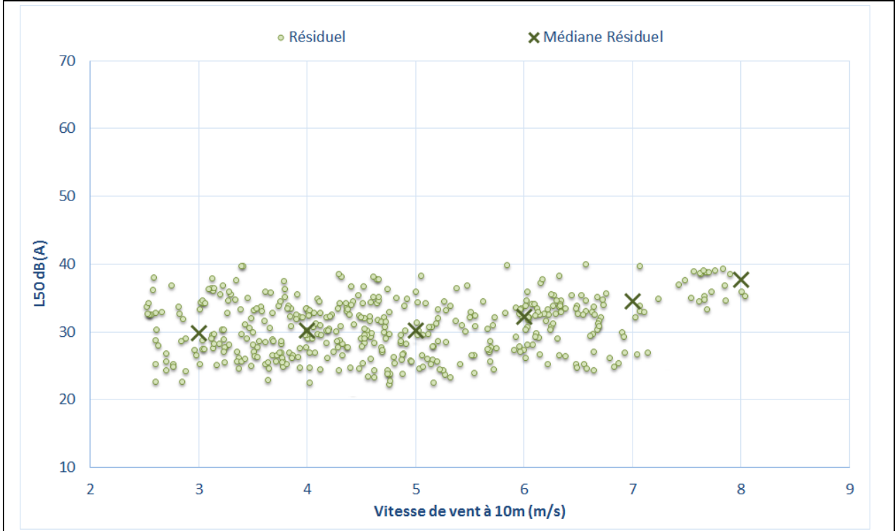
Figure 26 : Bruit en fonction de la vitesse de vent au point P5 – Mesures estivales
