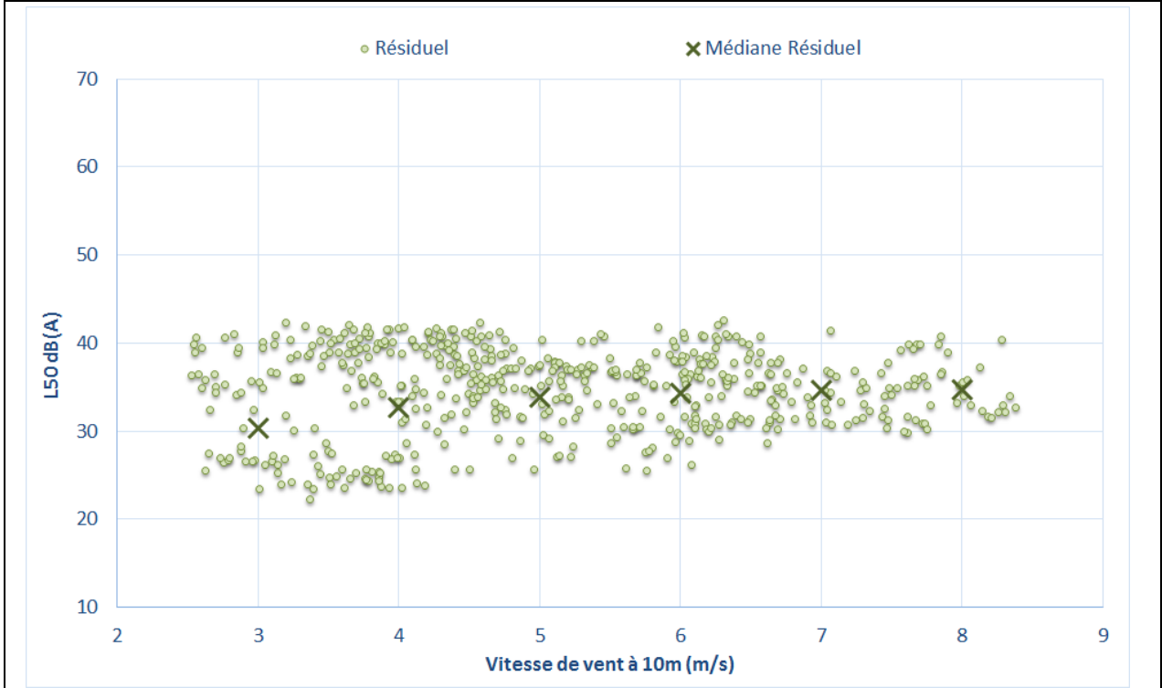
Figure 25 : Bruit en fonction de la vitesse de vent au point P4 – Mesures estivales
